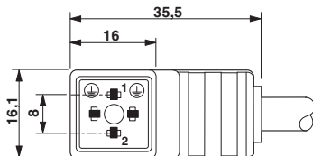
尺寸图
