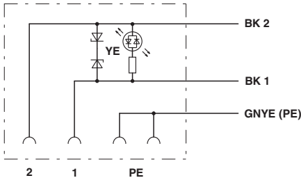
电路图
