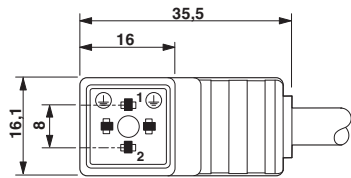
尺寸图
