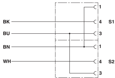
电路图
