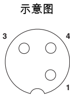
M12孔式连接器引分配，3芯，A编码，插座侧视图
