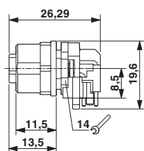
尺寸图
