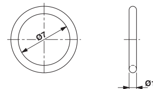
尺寸图
