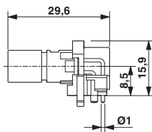
M12穿板式插拔连接器，针式，插芯，侧面视图
