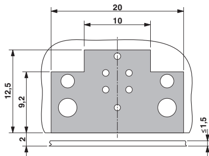
尺寸图
