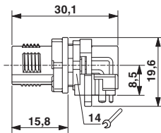
尺寸图
