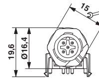
尺寸图
