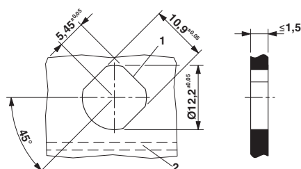
面板开口，PCB水平摆放(2)时的正面视图。第三个扁平区域为选配（1）。
