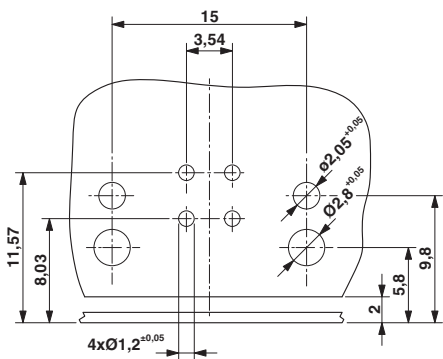
钻孔图
