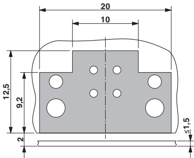
尺寸图
