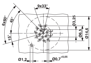
钻孔图
