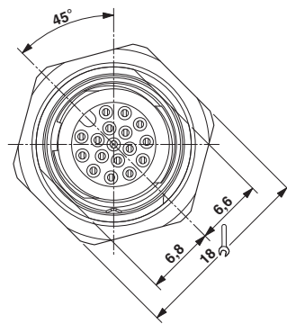
尺寸图
