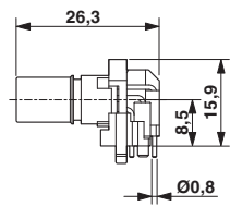
尺寸图
