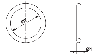
尺寸图
