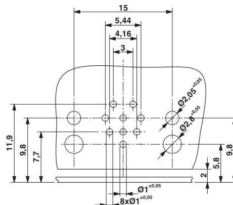
钻孔图
