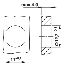
尺寸图
