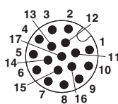
M12针式连接器的引脚分配，17芯，插头侧视图
