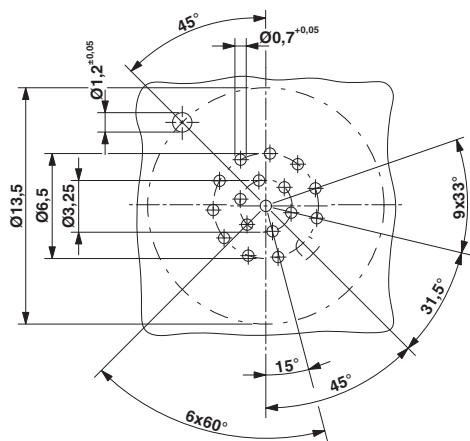
钻孔图
