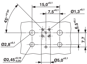
钻孔图
