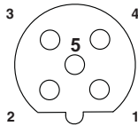
M12孔式连接器引脚分配，5芯，B编码，插座侧
