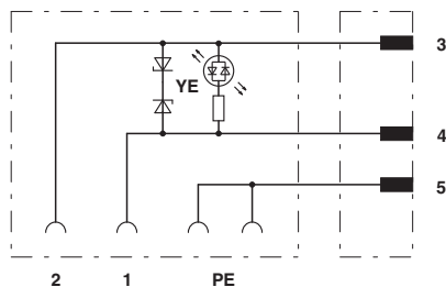
电路图
