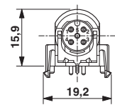
尺寸图
