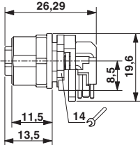
尺寸图
