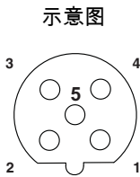
M12孔式连接器引脚分配，5芯，B编码，插座侧
