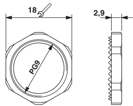
尺寸图
