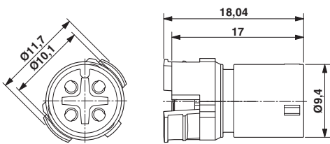
尺寸图
