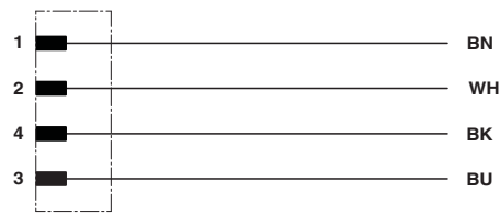
电路图
