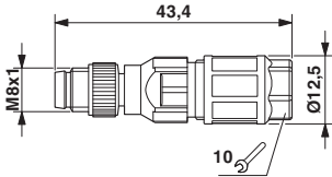
尺寸图
