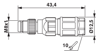
尺寸图
