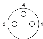
M8孔式引脚分配，3芯，插头侧视图
