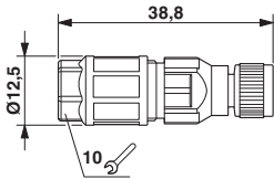
尺寸图
