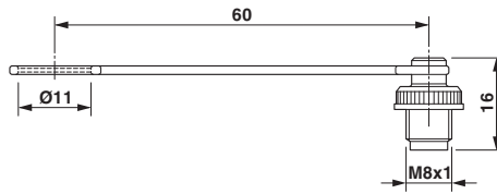
尺寸图
