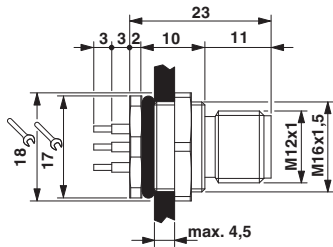
尺寸图
