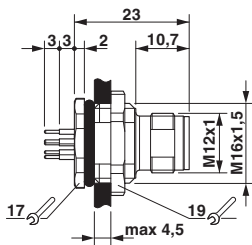
尺寸图
