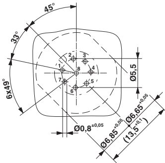
钻孔图
