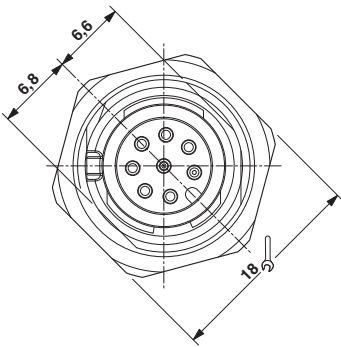
尺寸图
