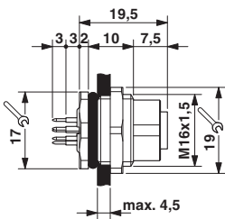
尺寸图
