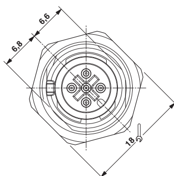
尺寸图
