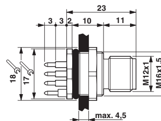
尺寸图
