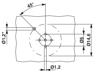
钻孔图
