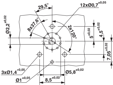
钻孔图
