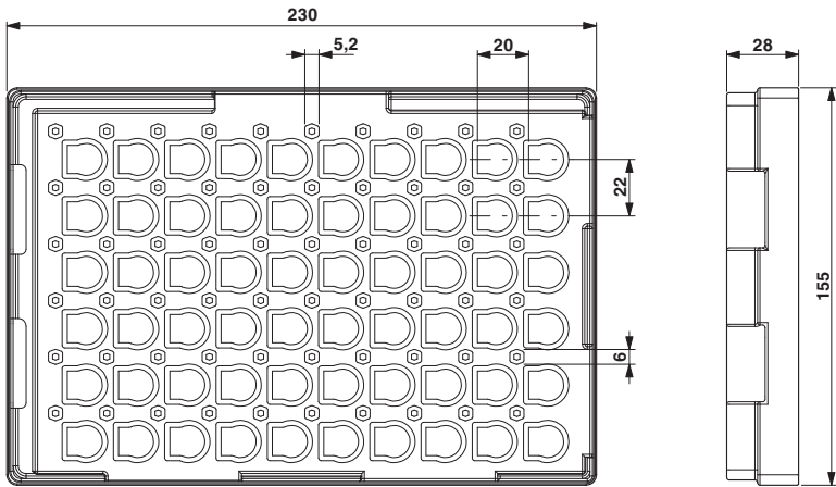
尺寸图
