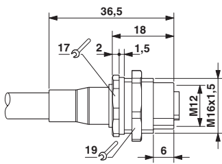
尺寸图
