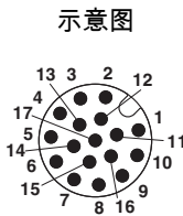
M12插头引脚分配，17芯，A编码，插头侧视图
