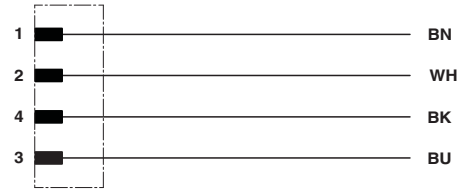
电路图
