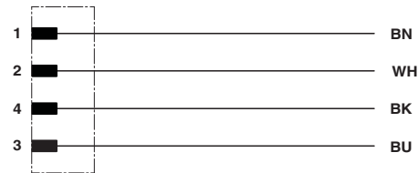
电路图
