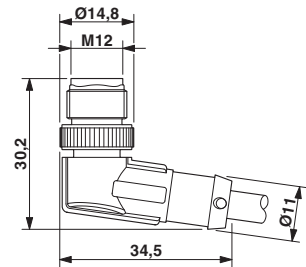
尺寸图
