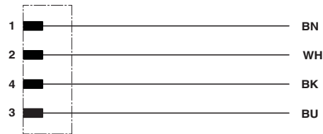
电路图
