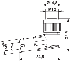
尺寸图
