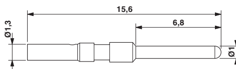
尺寸图
