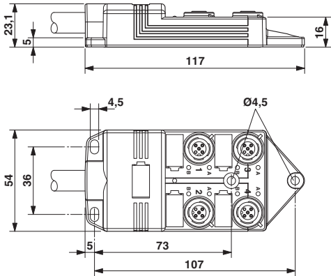
尺寸图
