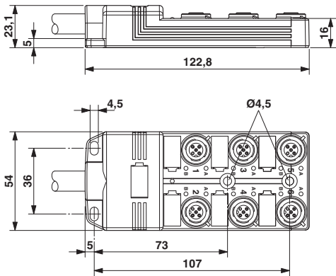
尺寸图
