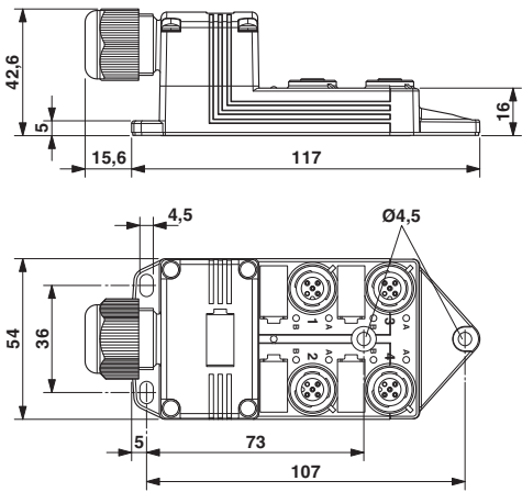
尺寸图
