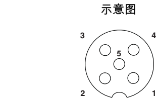
M12插槽，孔式，5芯
