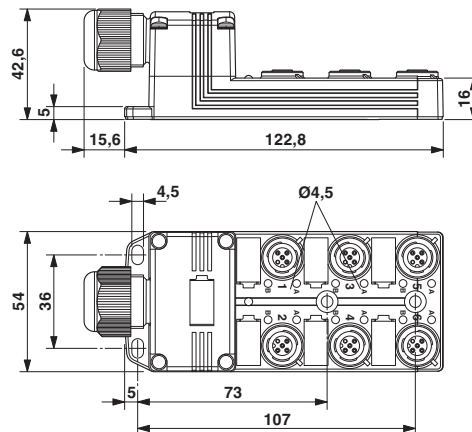
尺寸图
