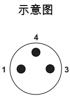
M8针式引脚分配，3芯，插头侧视图
