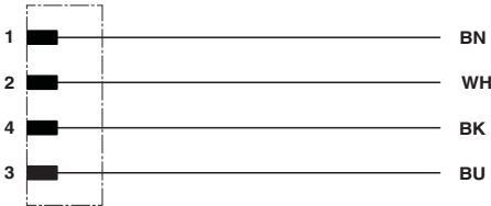
M8针式/孔式触点分配
