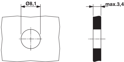
外壳开口，用于安装M8针式插座，一体式
