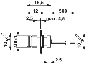
尺寸图
