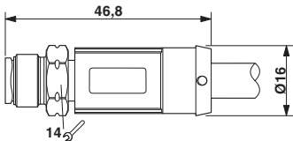
尺寸图
