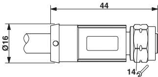
尺寸图
