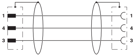
电路图
