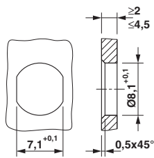
尺寸图
