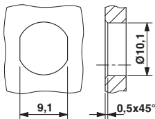
尺寸图
