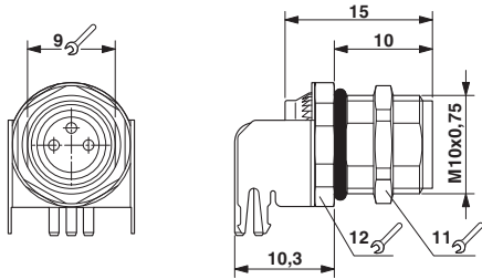
尺寸图
