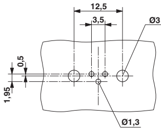
钻孔图
