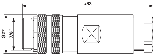
尺寸图
