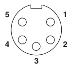
7/8"-16UNF孔式引脚分配，5芯，插座侧视图
