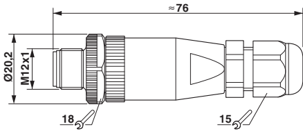
尺寸图
