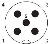
M12针式连接器引脚分配，5芯，A编码，插头侧
