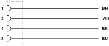
电路图
